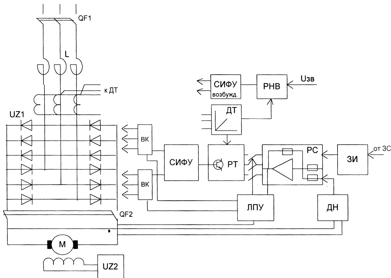
Рисунок 1 – Однолинейная схема электропривода механизмов крана
