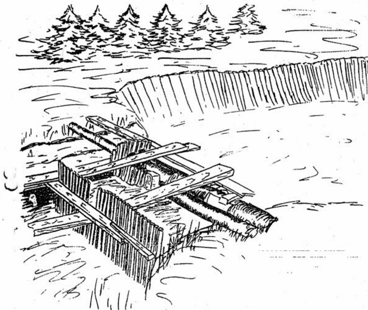
Рис. Естественный русловый садок для выдерживания производителей атлантического лосося.
