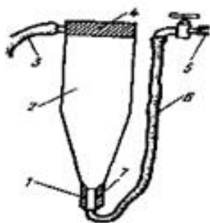
Рис. Аппарат Вейса: 1-металлическая трубка; 2-сосуд; 3-водосбрасывающий шланг; 4-железный обруч со сливным носиком; 5-водопроводный кран; 6-водопропадающий шланг; 7-пробка
