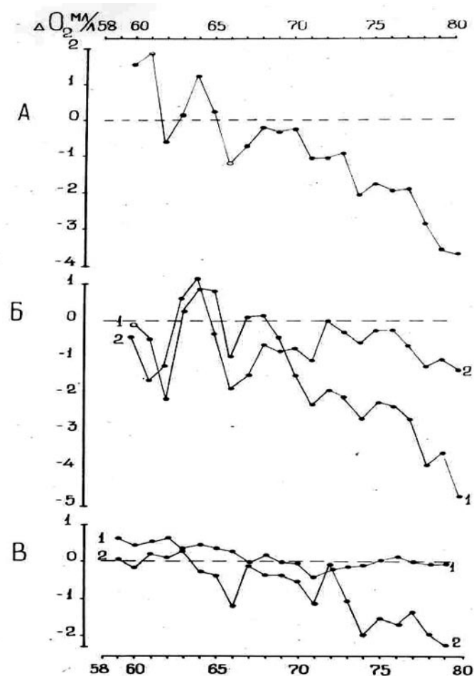
Рис. 2.26. Динамика трендов ( \Delta O_2 ) концентраций кислорода (мл/л) в придонном слое в летний сезон на северо-западном шельфе Черного моря с 1958 по 1980 г. [Фацук, 1985]. (Разрезы: А – Тендровская коса – Одесса; Б – Каркинитский залив – оз. Шаганы; В – мыс Тарханкут – Сулина.)
