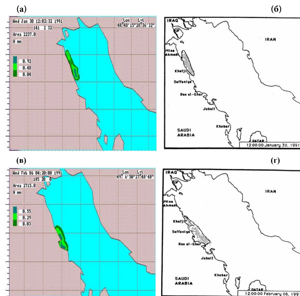
Рис. 4.6. Модельные расчеты динамики нефтяного пятна в Персидском заливе (а, в) и его фактическое положение по данным спутниковых наблюдений (б, г) [Овсиенко и др., 2005].
