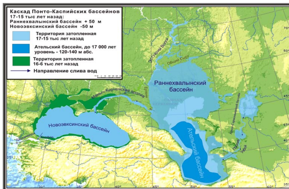
Рис. 1.16. Палеореконструкция связи Понто-Каспийских бассейнов в позднеледниковье и голоцене [Чепалыга, 2002]. 17–15 тыс. лет назад в результате потепления климата площадь Раннехвалынского бассейна (древнего Каспийского) увеличилась на 6 млн. км 2 , через Маньчж-Керченский пролив Каспий соединялся с Черным морем, а Аральское море через древний пролив Узбой соединялось с Каспием.
