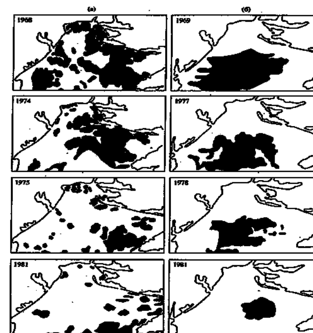
Рис. 3.10. Деградация площадей мидийных банок (а) и полей филофоры (б) на северо-западном шельфе Черного моря в результате развития здесь летних анаэробных зон [Фашук, 1995].
