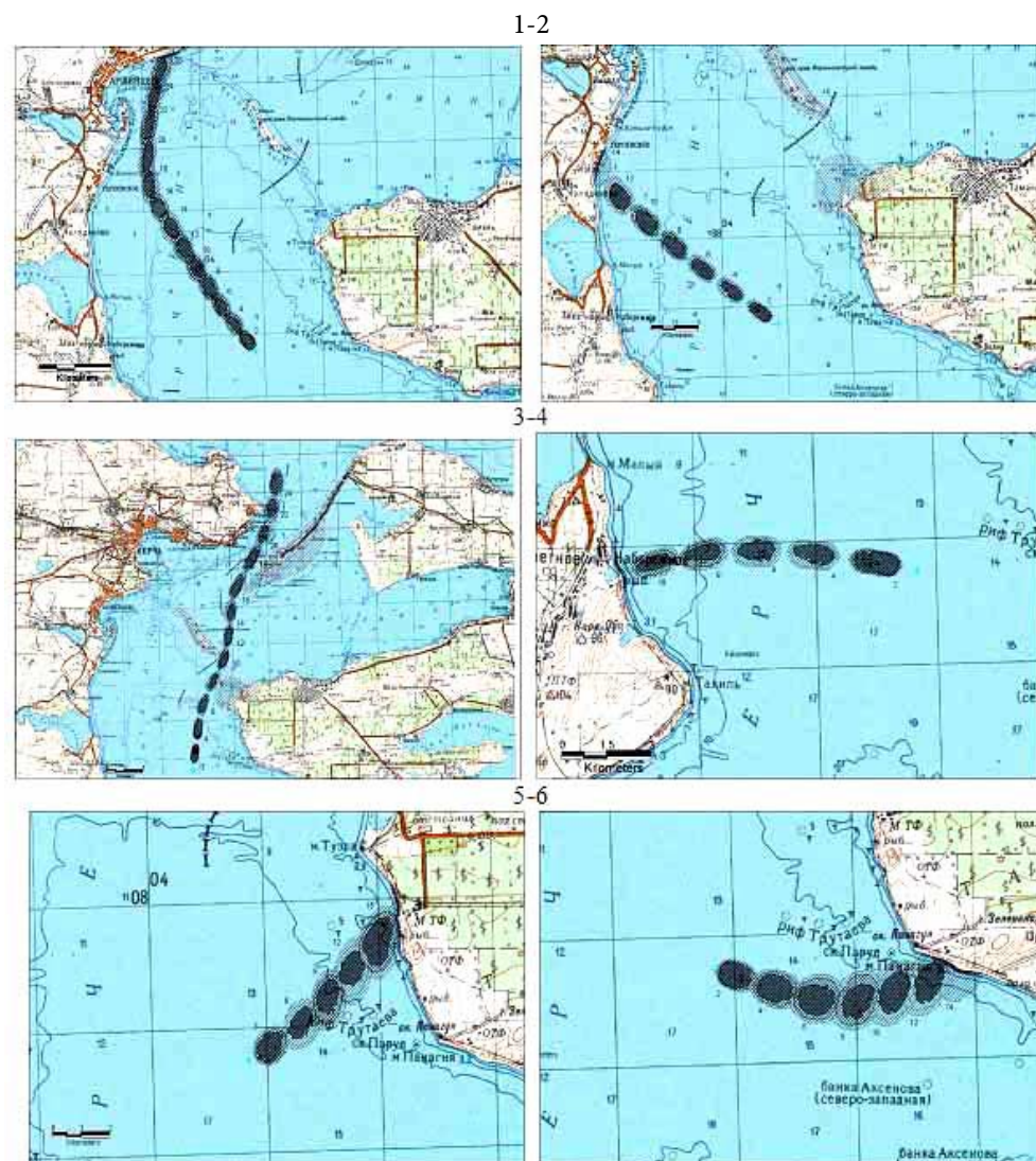
Рис. 3.18. Прогностическая динамика пятна сырой нефти после разлива (1500 т) на якорной стоянке у входа в Керченский пролив под влиянием преобладающих течений и конкретных ветровых ситуаций. Цифры у пятен – время после разлива. Траектории нефтяного разлива: 1, 2 – восточный ветер 5 и 10 м/с соответственно при черноморском потоке; 3 – южный ветер 10 м/с при черноморском потоке; 4 – восточный ветер 10 м/с при азовском потоке; 5 – западный ветер 10 м/с при черноморском потоке; 8 – западный ветер 10 м/с при азовском потоке.
