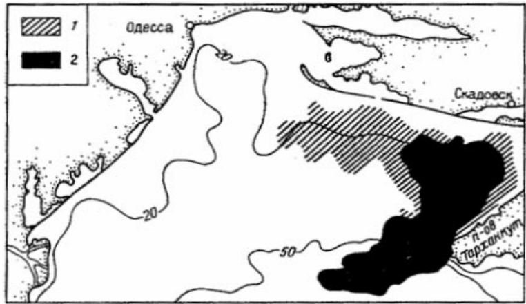
Рис. 3.13. Последствия донного тралового промысла и вторичного загрязнения для режима осадконакопления в северо-западной части Черного моря на период начала 80-х гг. [Зайцев, Фесюнов и др., 1992]. 1 – зона распространения мелкодисперсных частиц (наилка) в придонном слое (площадь – более 5 тыс. км 2 , скорость седиментации – 5–40 мм в год, на два-три порядка выше природной); 2 – зона с толщиной наилка 3–5 см (площадь – 3350 км 2 ), в том числе толщиной 30–50 см (площадь – 750 км 2 ).
