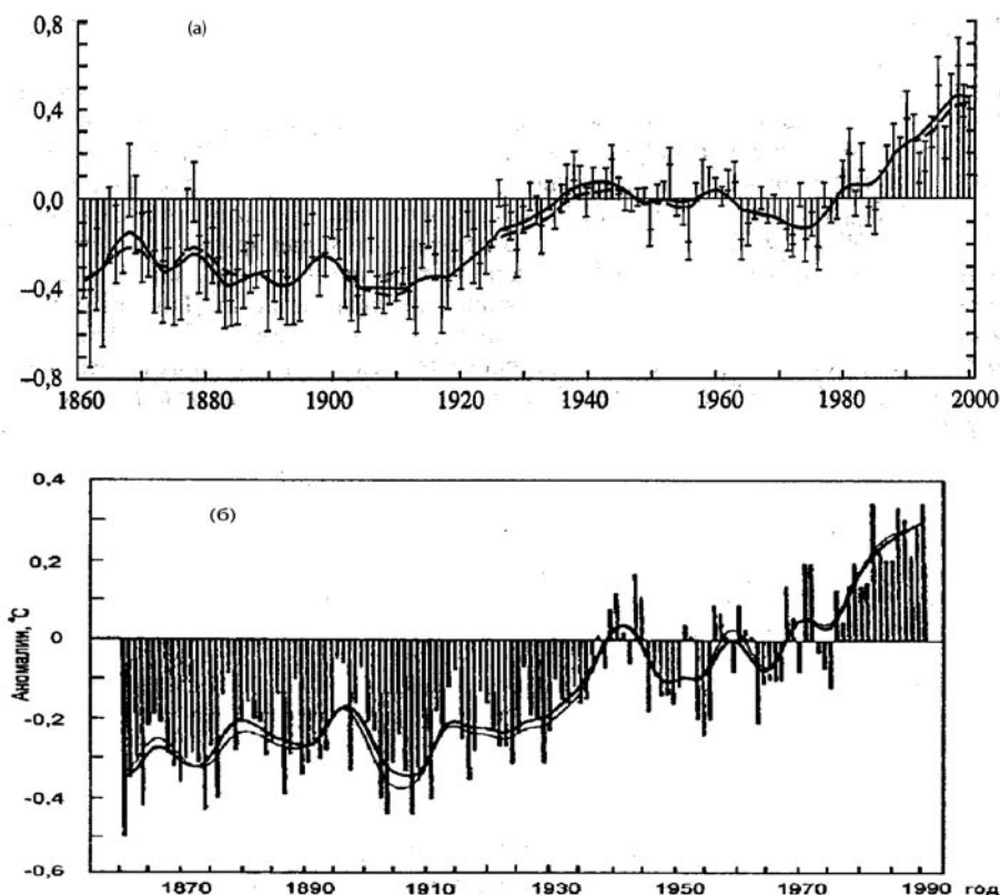
Рис. 1.8. Аномалии среднегодовой температуры воздуха в Северном (а) и Южном (б) полушариях за период 1860–2000 гг.
