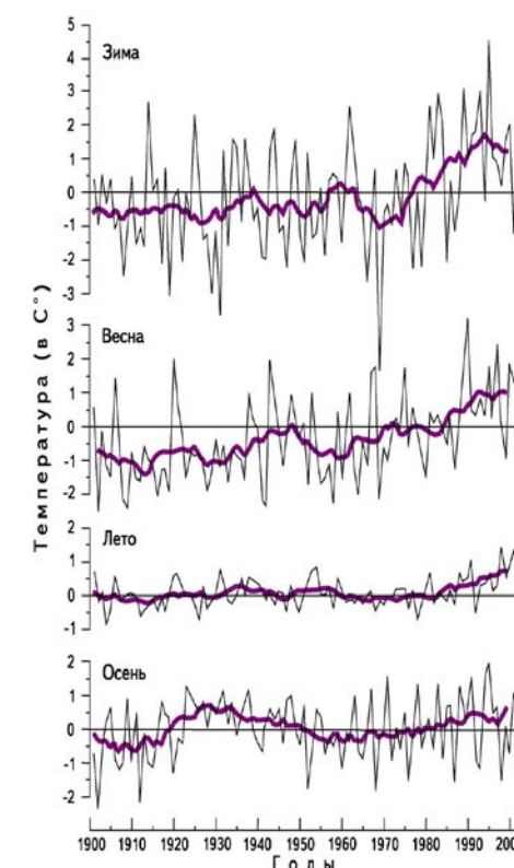
Рис. 1.10. Средние сезонные аномалии температуры воздуха на территории России за период 1901–2004 гг. [Национальный атлас..., 2008].
