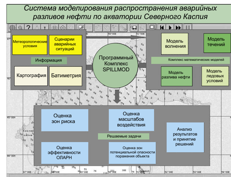
Рис. 4.2. Схема модельного комплекса «SPILLMOD» для условий Каспийского моря [Овсиенко и др., 2005].
