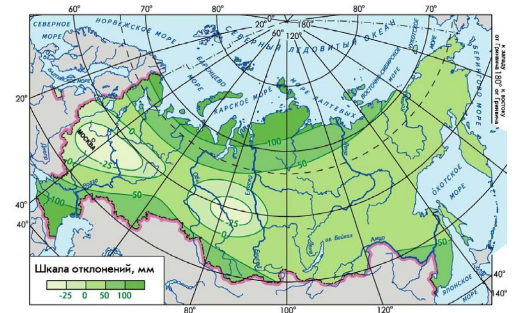
Рис. 1.11. Аномалии среднегодовой суммы осадков на территории России [Национальный атлас..., 2008].
