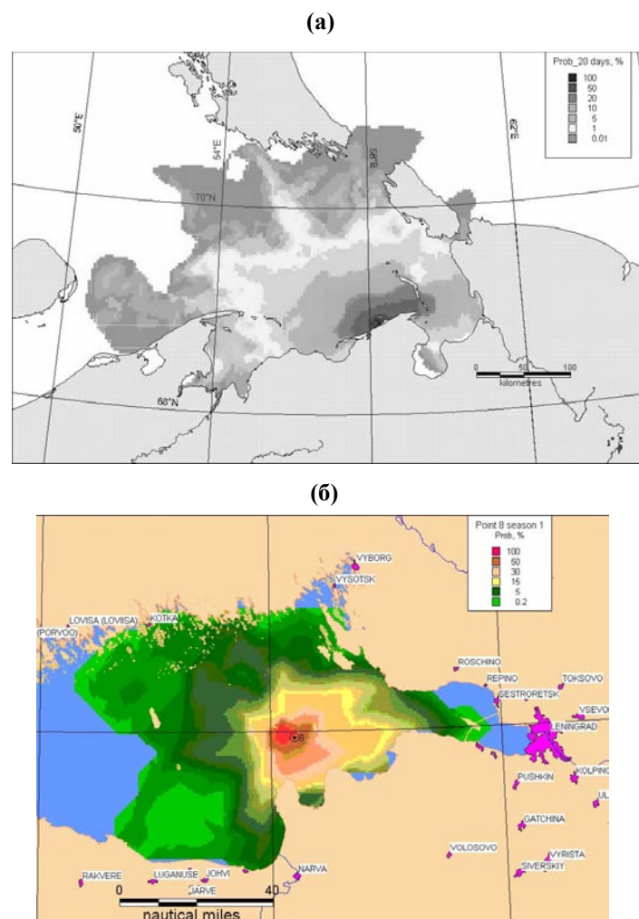
Рис. 4.5. Вероятность поражения нефтяным разливом участков акватории в районе терминала Варандей в Печорском море (а) и в зоне гипотетического разлива в Балтийском море (б) [Овсиенко и др., 2005].
