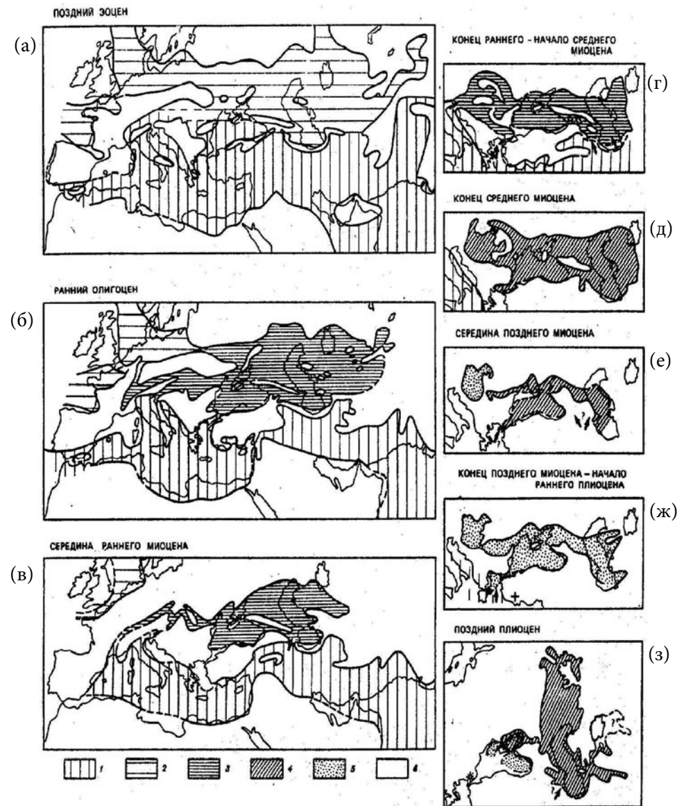
Рис. 3.2. Палеогеографические схемы Паратетиса и смежных бассейнов [Невеская и др., 1984]. 1 – Тетис и Средиземноморье; 2 – бореальные бассейны. Бассейн Паратетис: 3 – морской, 4 – полуморской, 5 – солоновато-водный; 6 – пресноводный. Стрелки – вероятное сообщение Паратетиса с открытыми морскими бассейнами.
