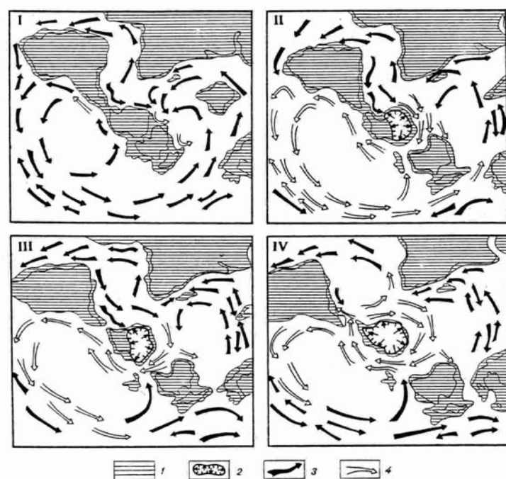
Рис. 1.1. Палеотечения в океанах Южного полушария [Котляков, 1994]. I – плиоцен (60 млн. лет назад);
