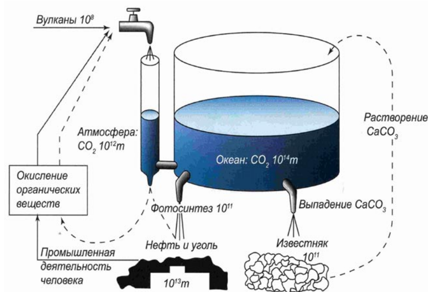
Рис. 1.3. Гидродинамическая модель обмена \text{CO}_2 между атмосферой и океаном по типу сообщающихся сосудов [Айзатулин и др., 1979].
