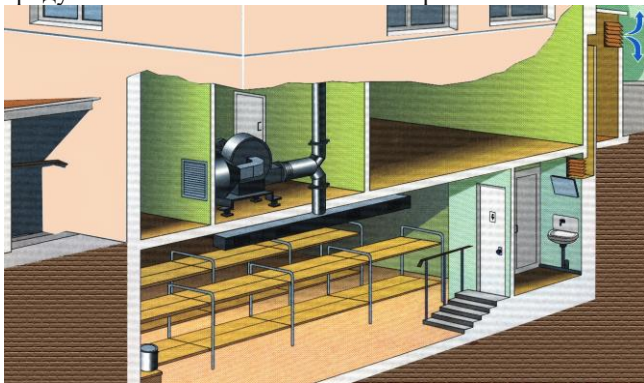
Рис. 3 — Противорадиационное укрытие
