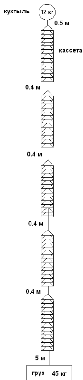
Рисунок 4.21. Схема оптимальной конструкции гирлянды коллекторов
