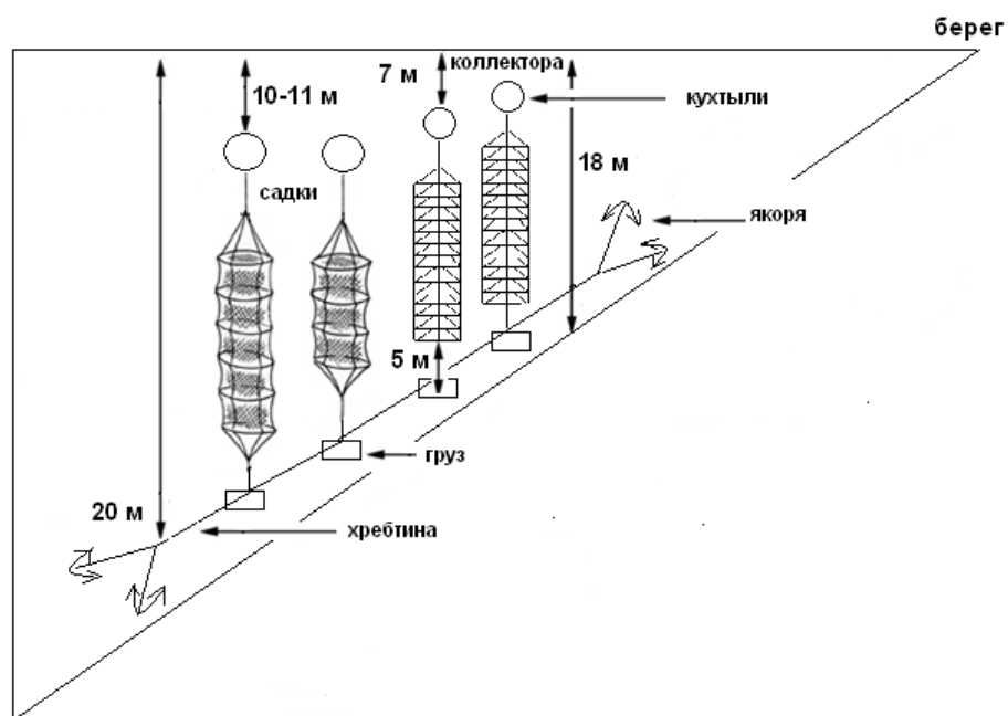
Рисунок 5.2. Схема постановки конструкций марикультуры для участка № 65-10-18 (залив Анива)
