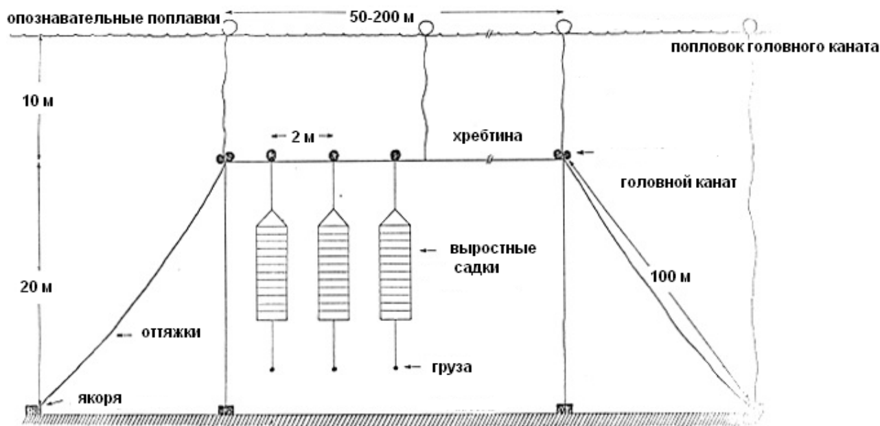
Рисунок 5.1. Схема постановки конструкций марикультуры, применяемая в странах азиатско-тихоокеанского региона.
